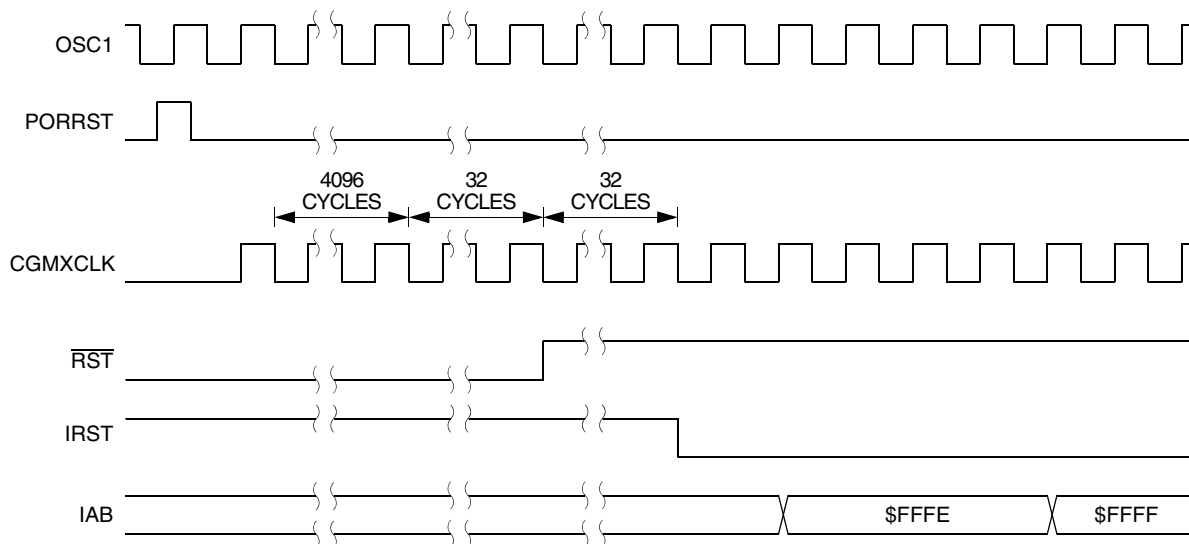
Figure 4-7. POR Recovery
