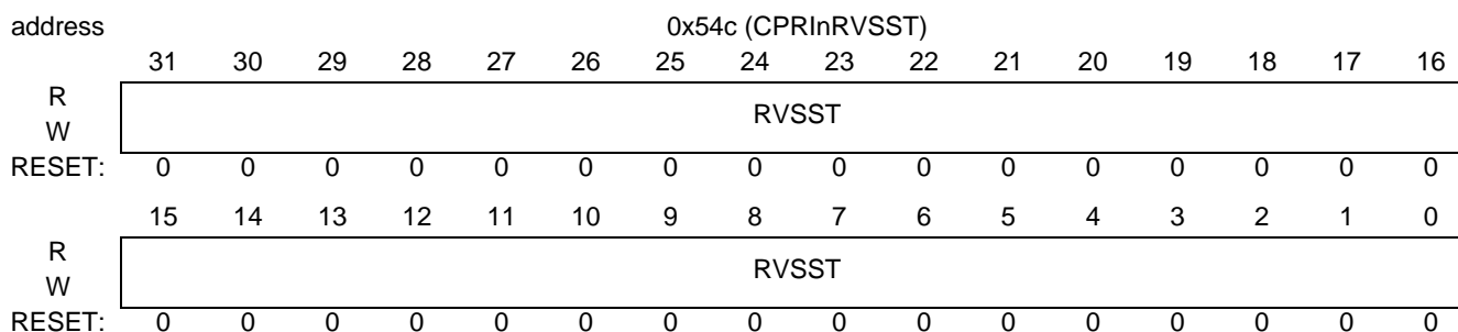
Figure 18-127. CPRInRVSST
