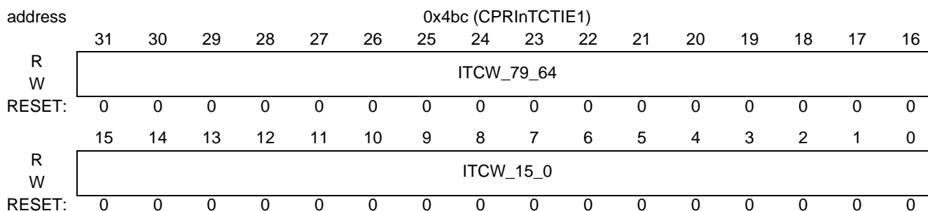
Figure 18-104. CPRInTCTIE1
